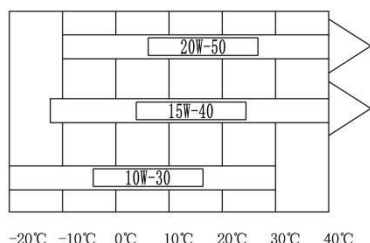
Рисунок 16 Выбор масла.
